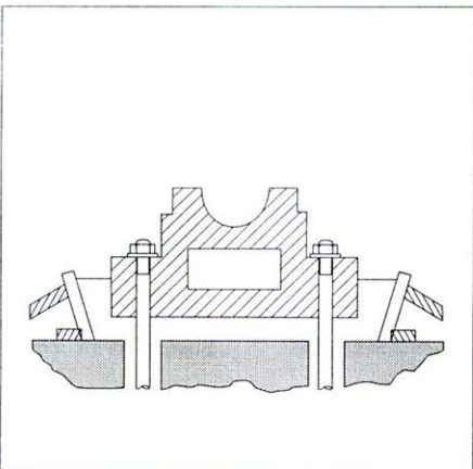
Zalijevanje temelja stroja
