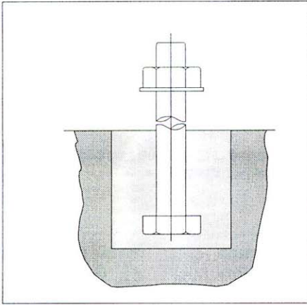
Usađivanje kotvi i klinova
