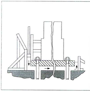
Zalijevanje temelja stroja
