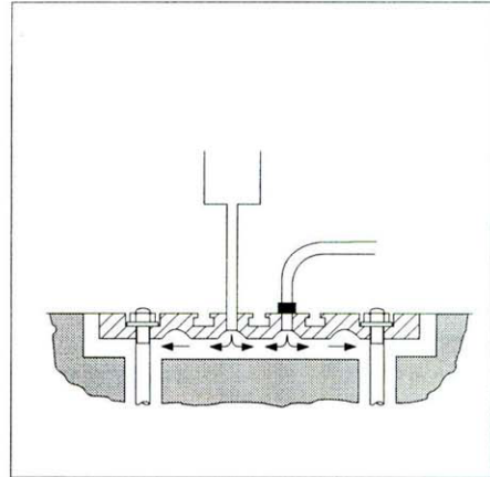
Podlijevanje neravnih temeljnih ploča
