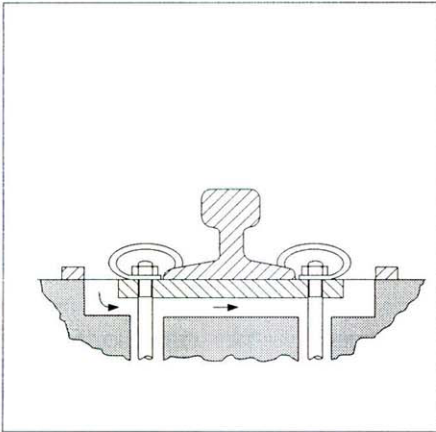
Podlijevanje kranskih šina
