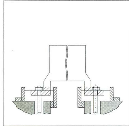
Zalijevanje strojeva sa razdjeljenim temeljnim pločama
